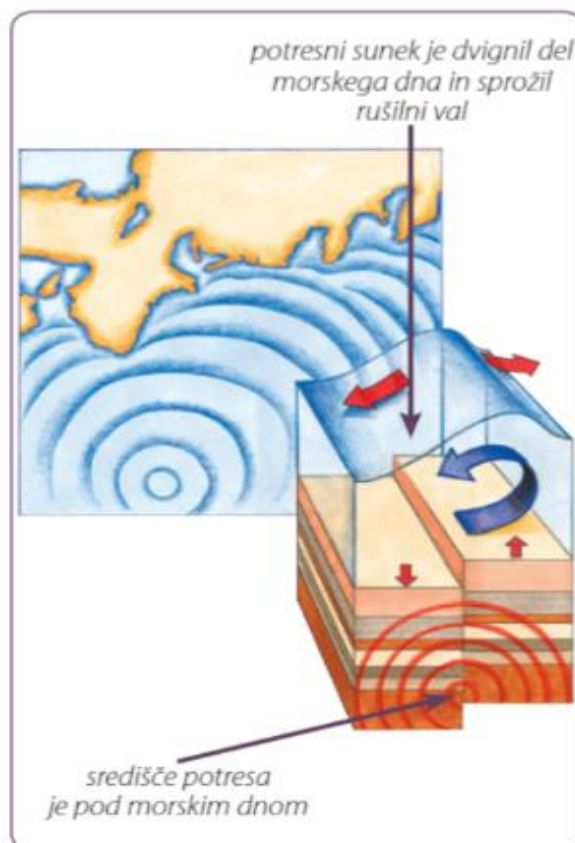
Nastanek cunamija
